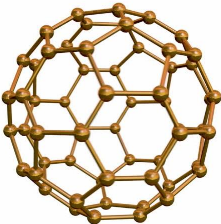
Молекула фуллерена
